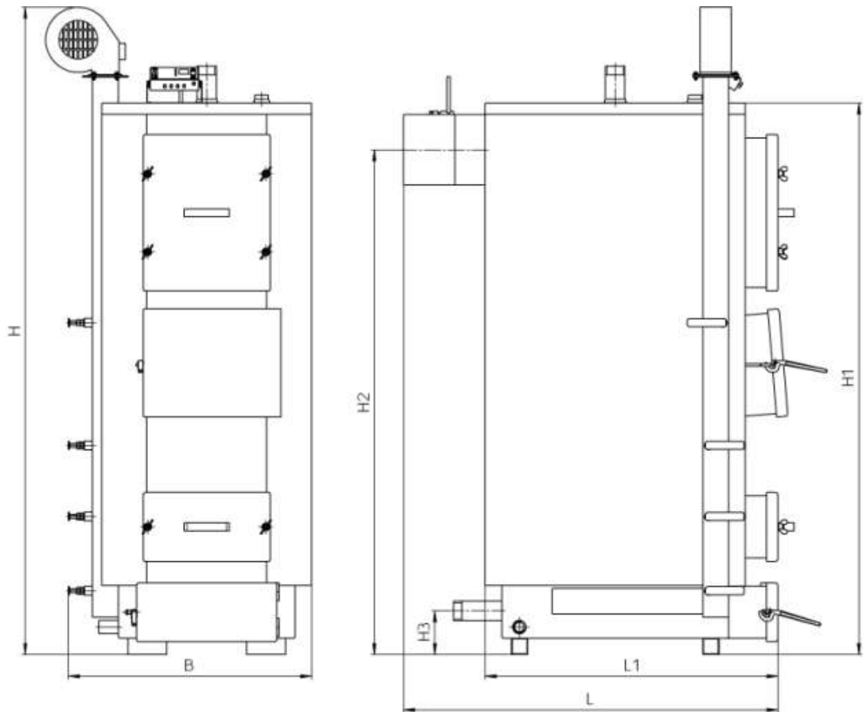
Рисунок 1 – Габаритне креслення котла типу КТ-2
