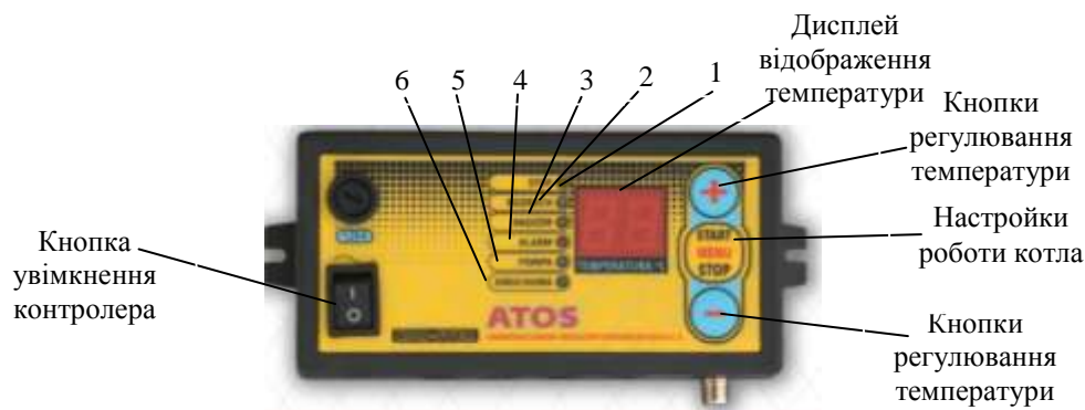
Рисунок 3 - Лицьова панель контролера
